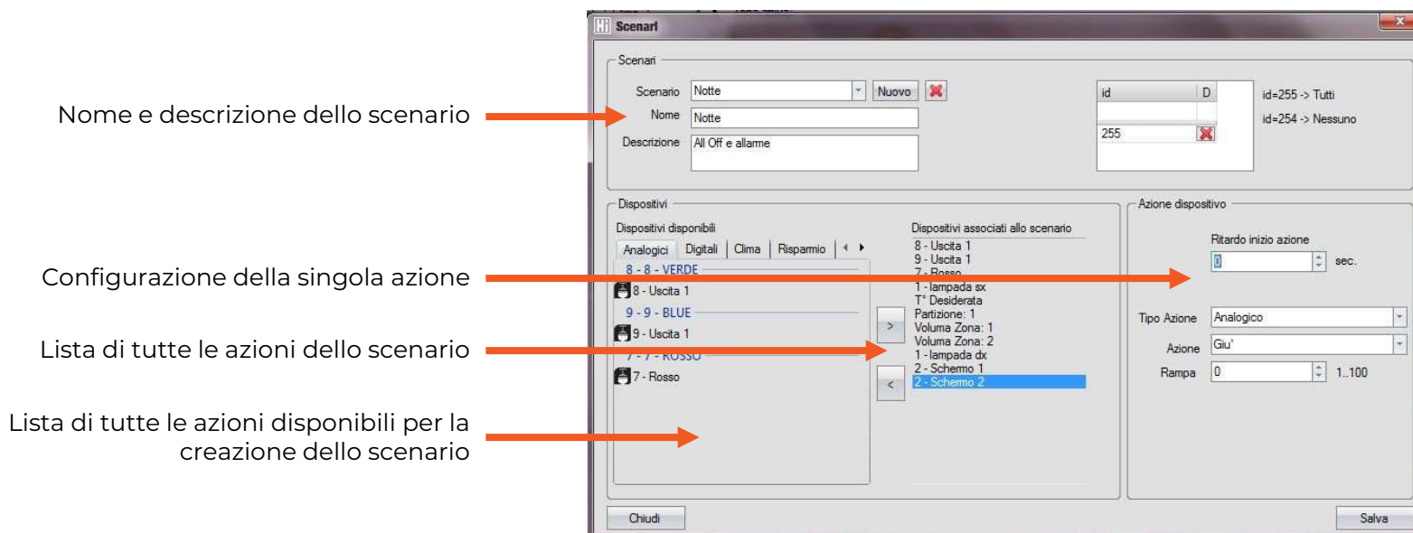
Figura 6: Strumento di creazione e gestione degli Scenari integrati
