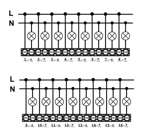
f Collegamento carichi (impiego EK-F11-TP come uscita binaria 16 canali)
