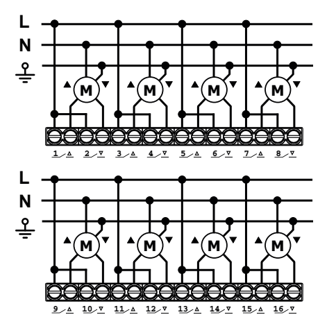
g Collegamento carichi (impiego EK-F11-TP come attuatore 8 canali per controllo di azionamenti)
