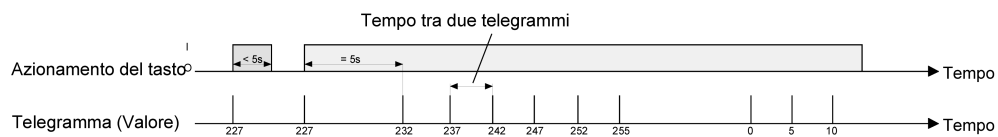
Figura 39: Esempio per la regolazione del valore con sovracorsa del campo di valori
