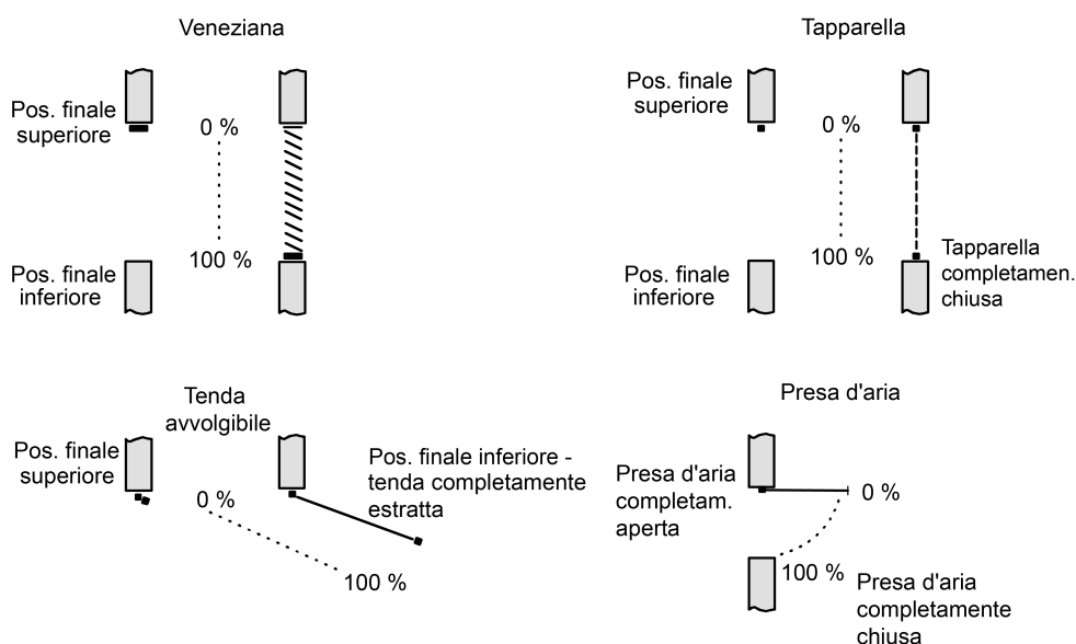
Figura 9: Definizione della posizione secondo il tipo di azionamento
