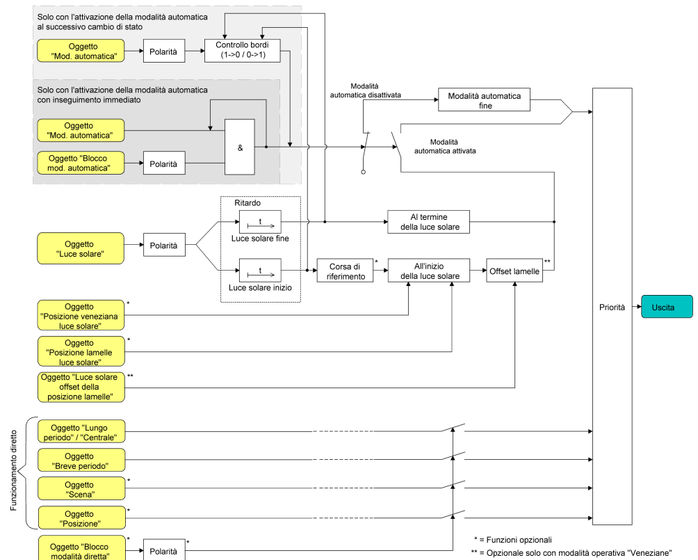
Figura 17: Schema elettrico funzionale della protezione contro il sole avanzata
