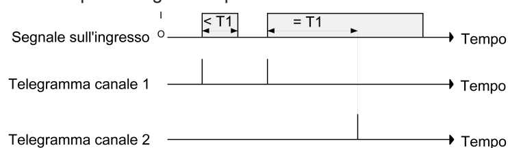
Figura 45: Esempio della procedura di comando "Canale 1 e canale 2"
