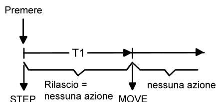
Figura 36: Procedura di comando: "Breve - Lungo"
