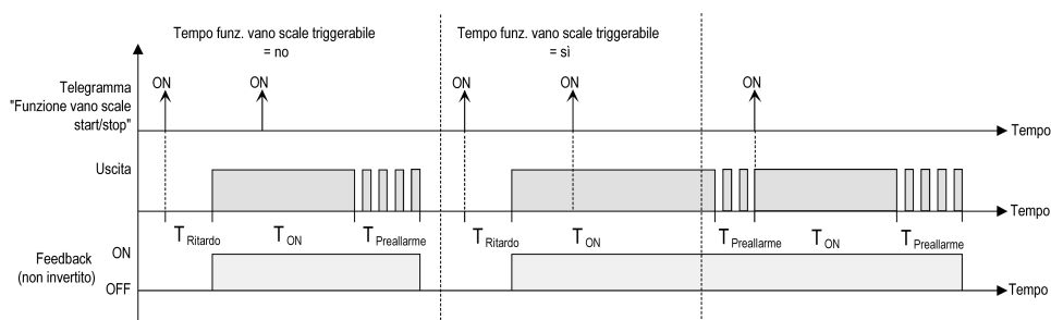
Figura 24: Comportamento di attivazione della funzione vano scale
