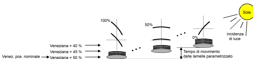
Figura 10: Esempio di posizionamento delle lamelle con effetto sulla posizione della veneziana
