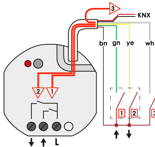
Figura 30: Modalità di funzionamento degli ingressi in caso di comando dell'uscita veneziana interna
