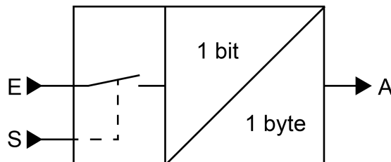
Figura 46: Convertitore (1 Bit -> 1 Byte)
