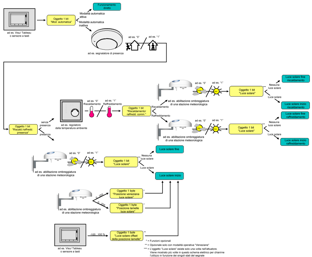
Figura 19: Schema elettrico di principio riscaldamento/raffreddamento in automatico
