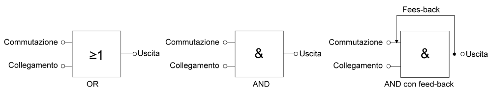
Figura 28: Tipi di collegamento della funzione logica
