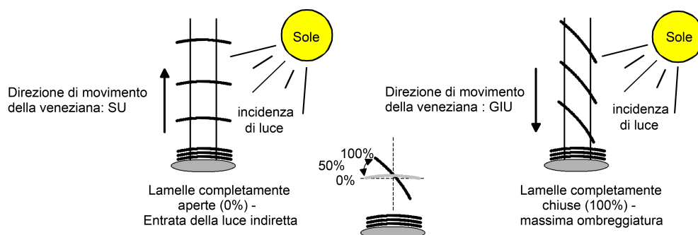
Figura 8: Tipo 2 - Veneziane a lamelle con posizione inclinata e diritta delle lamelle
