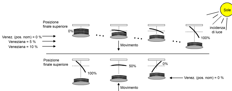
Figura 11: Esempio di posizionamento delle lamelle con veneziana in posizione finale superiore (Esempio per lamelle di tipo 1.)
