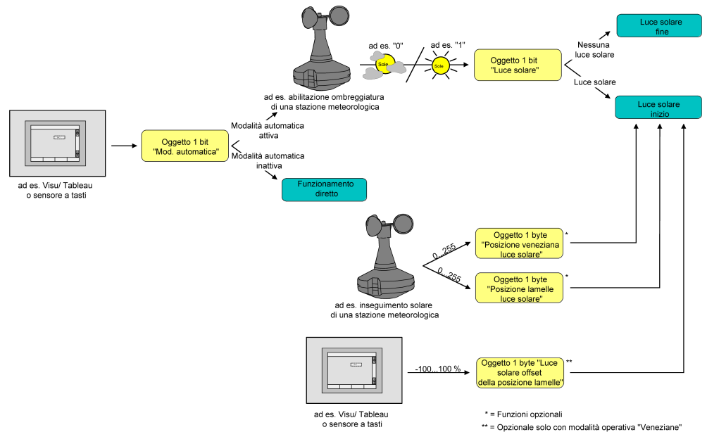
Figura 16: Schema elettrico di principio della protezione contro il sole avanzata (per semplicità senza funzioni di blocco)
