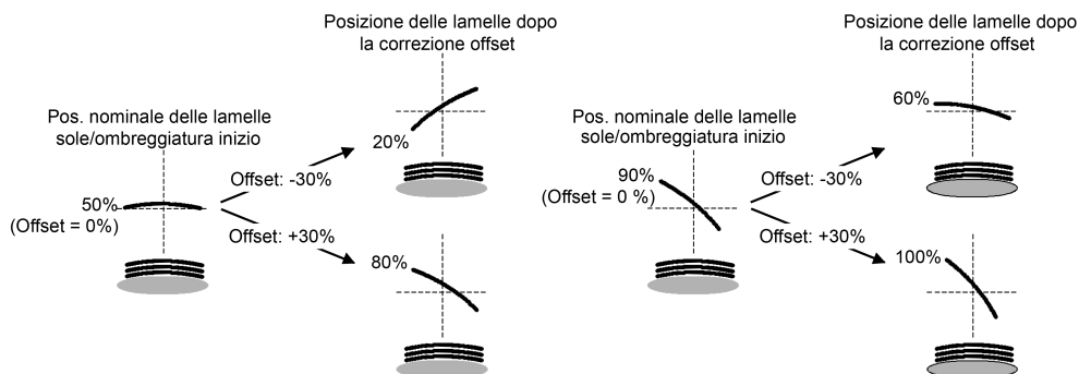
Figura 18: Esempio della modalità di funzionamento dell'offset lamelle (esempio per il tipo di lamelle 1 / il tipo di lamelle 2 è analogo)
