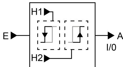
Figura 49: Interruttore del valore limite
