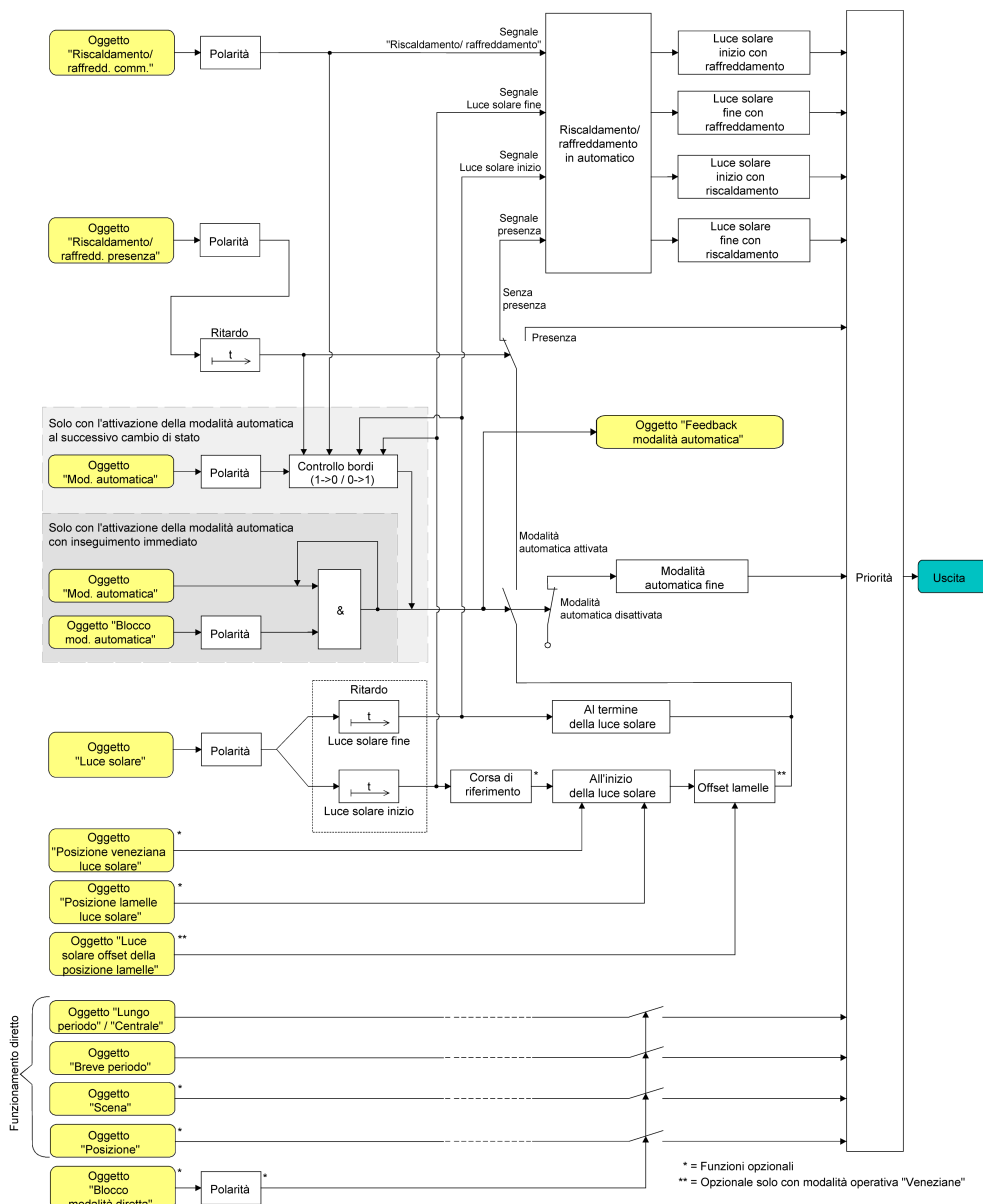
Figura 20: Schema elettrico funzionale riscaldamento/raffreddamento in automatico
