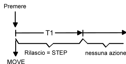
Figura 35: Procedura di comando "Lungo - Breve"
