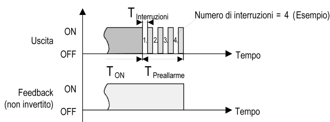
Figura 26: Funzione di preavvertimento della funzione vano scale (esempio)
