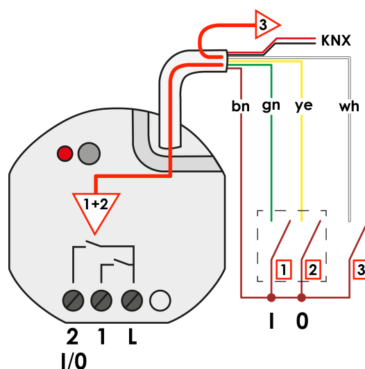
Figura 33: Modalità di funzionamento degli ingressi in caso di comando dell'uscita di commutazione interna 2 come comando a due pulsanti
