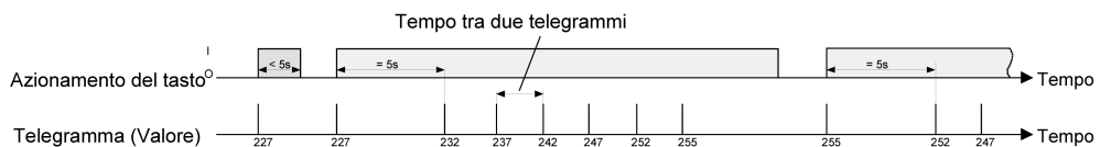
Figura 38: Esempio per la regolazione del valore senza sovracorsa del campo di valori
