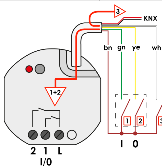
Figura 32: Modalità di funzionamento degli ingressi in caso di comando dell'uscita di commutazione interna 1 come comando a due pulsanti
