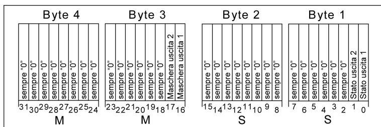
Figura 23: Struttura dell'oggetto del feed-back cumulativo
