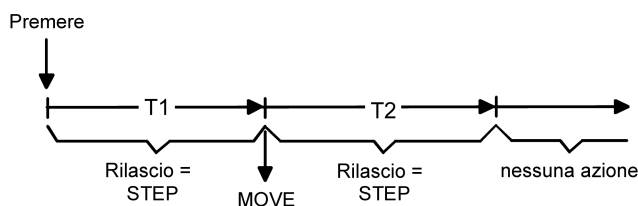
Figura 37: Procedura di comando "Lungo – Breve o Breve"
