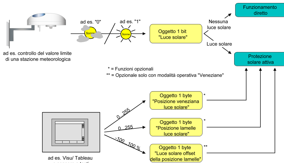
Figura 14: Schema elettrico di principio della protezione contro il sole semplice
