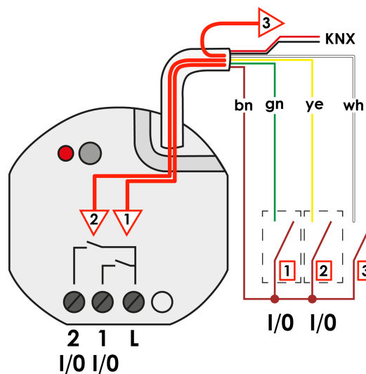
Figura 31: Modalità di funzionamento degli ingressi in caso di comando delle uscite di commutazione interne come comando a un pulsante
