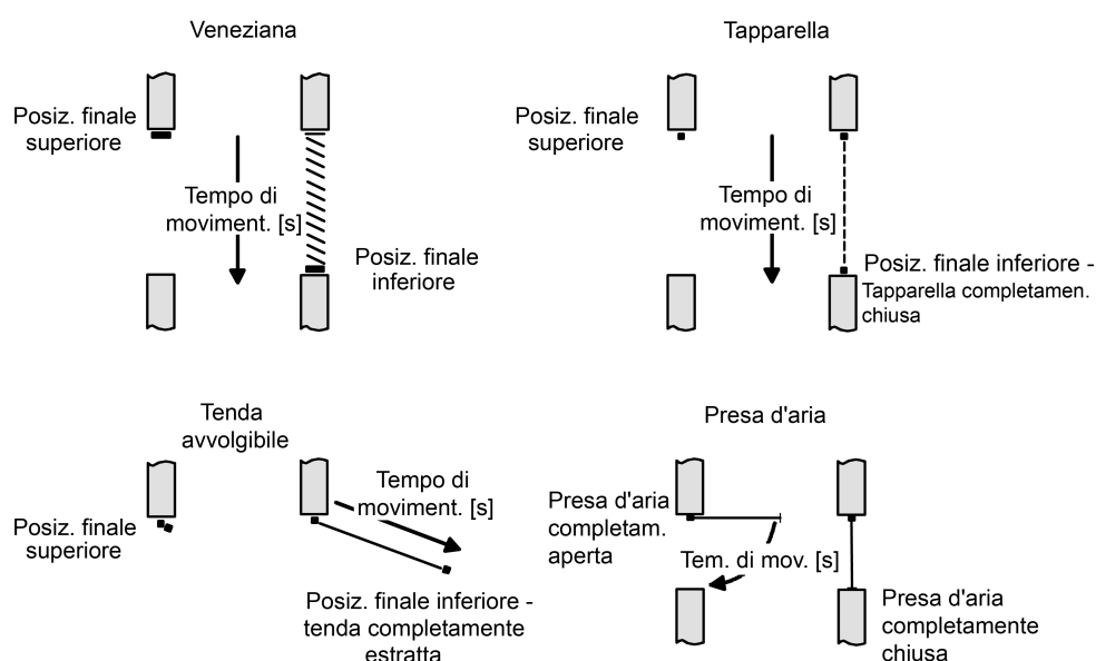
Figura 6: Determinazione del tempo di movimento secondo il tipo di azionamento
