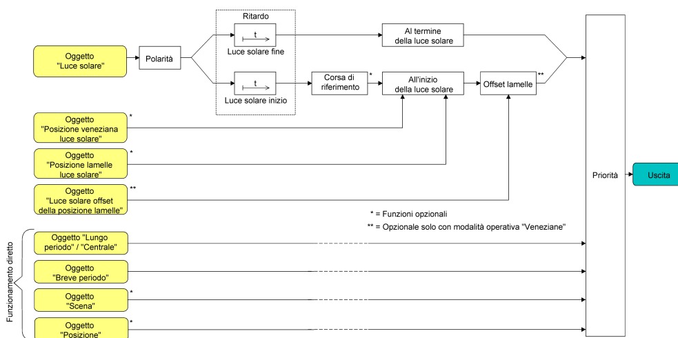
Figura 15: Schema elettrico funzionale della protezione contro il sole semplice
