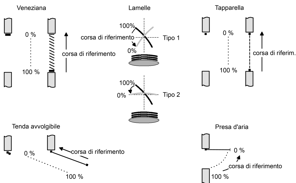
Figura 12: Corsa di riferimento
