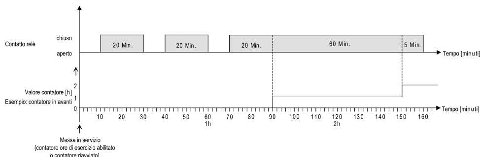
Figura 29: Funzionamento del contaore (esempio di ore conteggiate)
