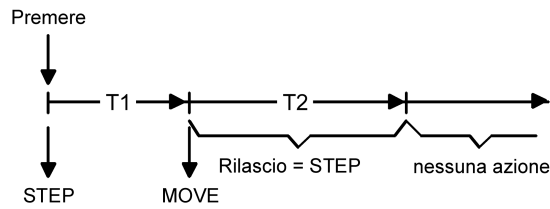
Figura 34: Procedura di comando "Breve - Lungo - Breve"
