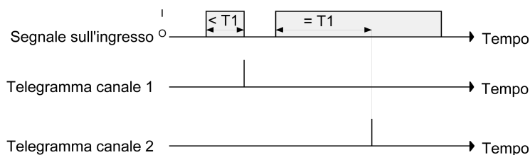
Figura 44: Esempio della procedura di comando "Canale 1 o canale 2"
