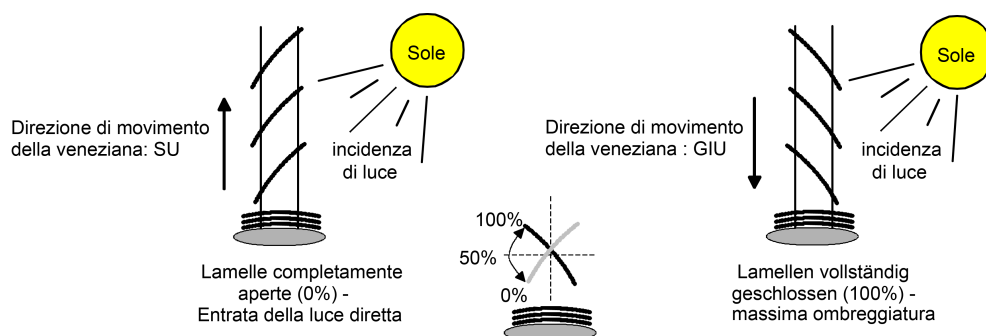
Figura 7: Tipo 1 - Veneziane a lamelle con posizione inclinata delle lamelle in entrambi i sensi di movimento
