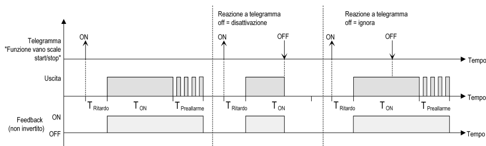
Figura 25: Comportamento di disattivazione della funzione vano scale
